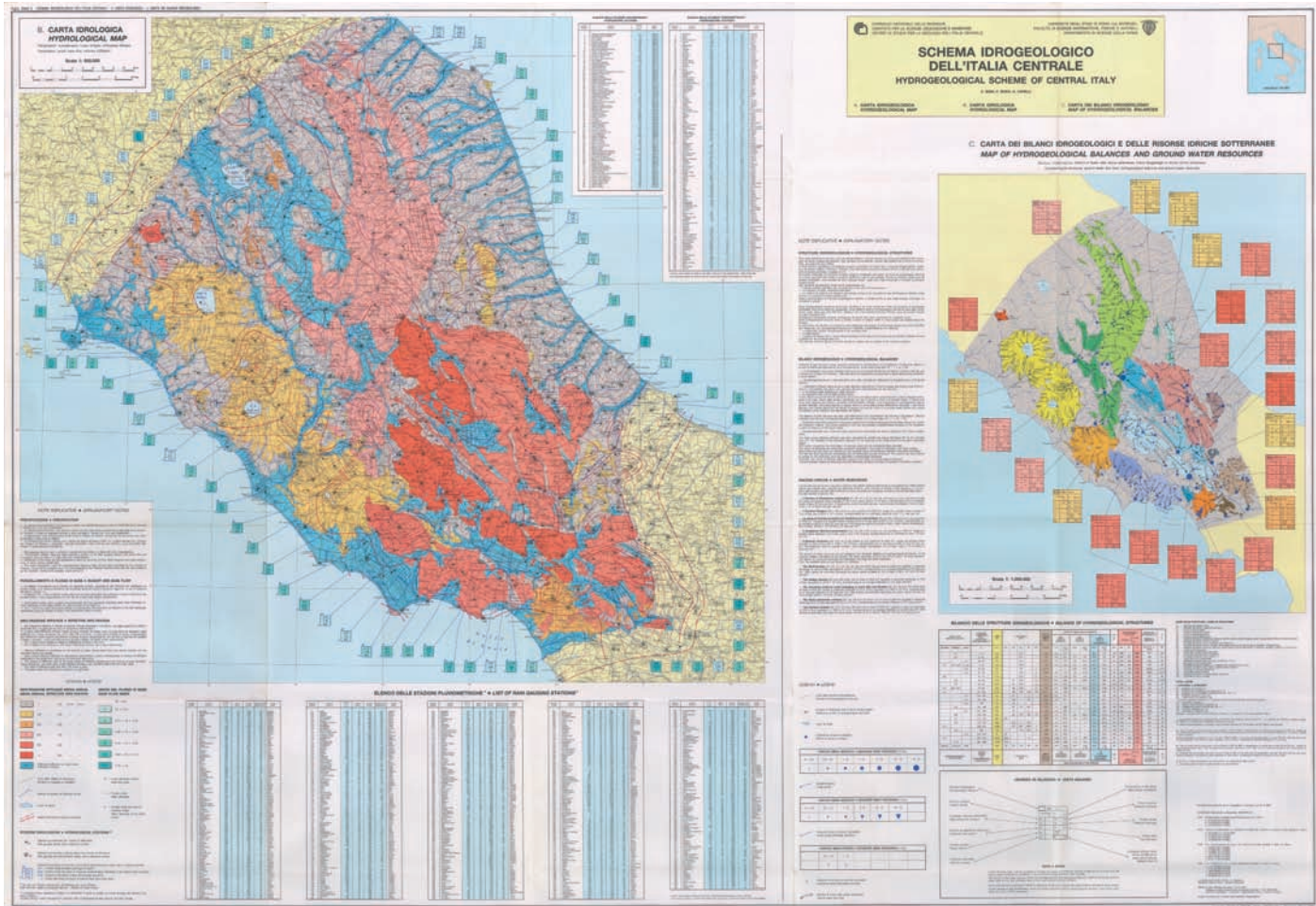
Fig. 2 - Schema Idrogeologico dell'Italia centrale (foglio 2) - Carta Idrologica (B) (scala 1:500.000) e Carta dei bilanci idrogeologici e delle risorse idriche sotterranee (C) (scala 1:1.000.000) (BONI et alii , 1986) - Hydrogeological sketch of central Italy (sheet 2) - Hydrological map (B) (1:500,000) and Map of hydrogeological balances and groundwater resources (C) (1:1,000,000) (BONI et alii , 1986)
