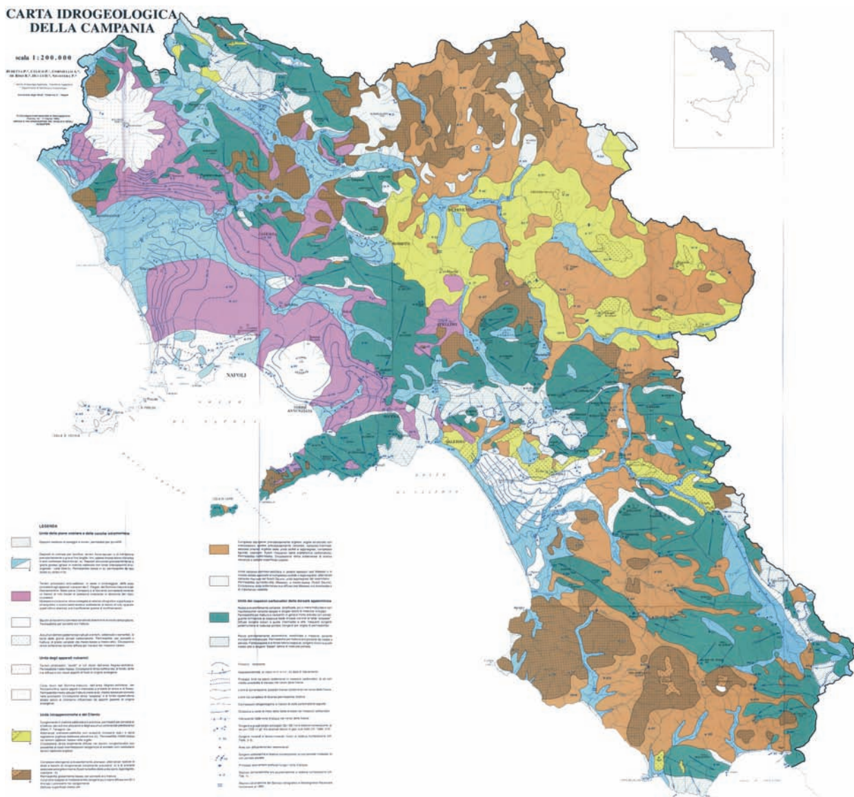
Fig. 9 - Carta idrogeologica della Campania (scala 1:200.000) (BUDETTA et alii , 1994) - Hydrogeological map of Campania (1:200.000) (BUDETTA et alii , 1994)
