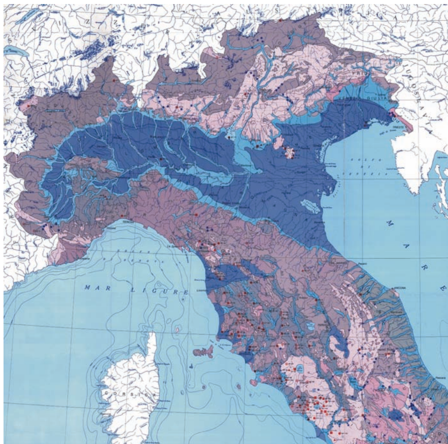
Fig. 5 - Carta delle manifestazioni termali e dei complessi idrogeologici d'Italia - Foglio nord (scala 1:1.000.000) (BONI et alii , 1982) - Map of Italian thermal manifestations and hydrogeological complexes - Sheet of northern Italy (1:1,000,000) (BONI et alii , 1982)
