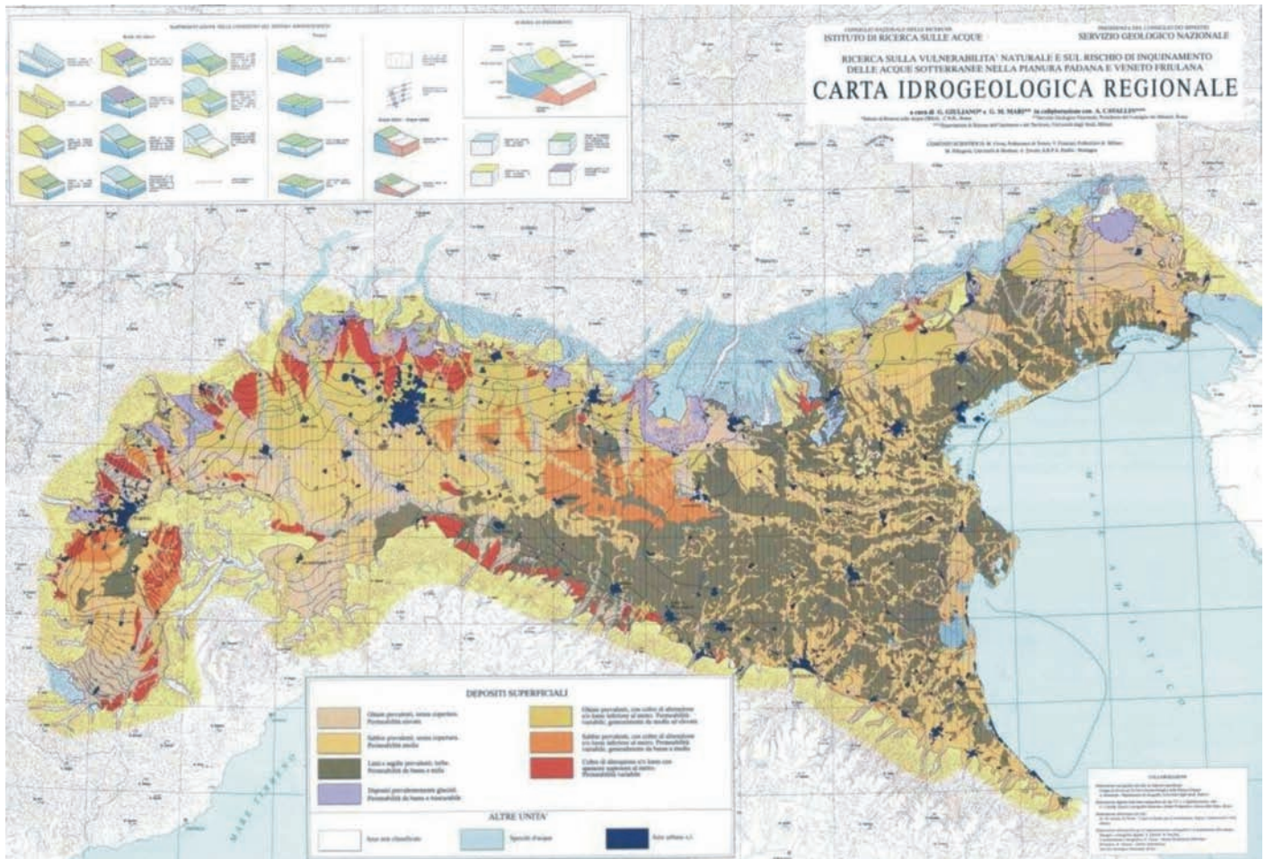
Fig. 10 - Ricerca sulla vulnerabilità naturale e sul rischio di inquinamento delle acque sotterranee della Pianura Padana e Veneto-Friulana - Carta idrogeologica regionale (scala 1:500.000) (GIULIANO et alii , 1998) - Research on natural vulnerability and groundwater pollution risk in the Po River and Veneto-Friuli valleys - regional hydrogeological map (1:500.000) (GIULIANO et alii , 1998)
