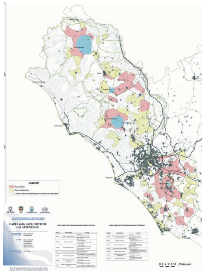
Fig. 7 - Uso compatibile della risorsa idrica degli acquiferi vulcanici del Lazio - Carta delle Aree Critiche e di Attenzione (scala 1:200.000) (CAPELLI et alii , 2005) - Sustainable use of water resources from the volcanic aquifers of Lazio - Map of Critical and Attention Areas (scale 1:200.000) (CAPELLI et alii , 2005)
