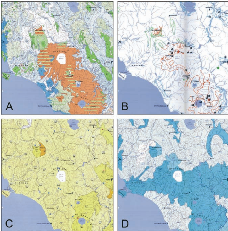
Fig. 4 - Studio sulle risorse in acque sotterranee in Italia - A: stralcio della carta delle formazioni acquifere; B: stralcio della carta dell'idrologia sotterranea; C: stralcio della carta dei prelievi; D: stralcio della carta della valutazione delle disponibilità residue (scala 1:500.000) (COMMISSIONE DELLE COMUNITÀ EUROPEE, 1982) - Study on Italian groundwater resources - A: excerpt from map of aquiferous formations; B: excerpt of subsurface hydrology map; C: excerpt of withdrawal map; D: excerpt of residual availability map (scale 1:500.000) (COMMISSION OF THE EUROPEAN COMMUNITIES, 1982)
