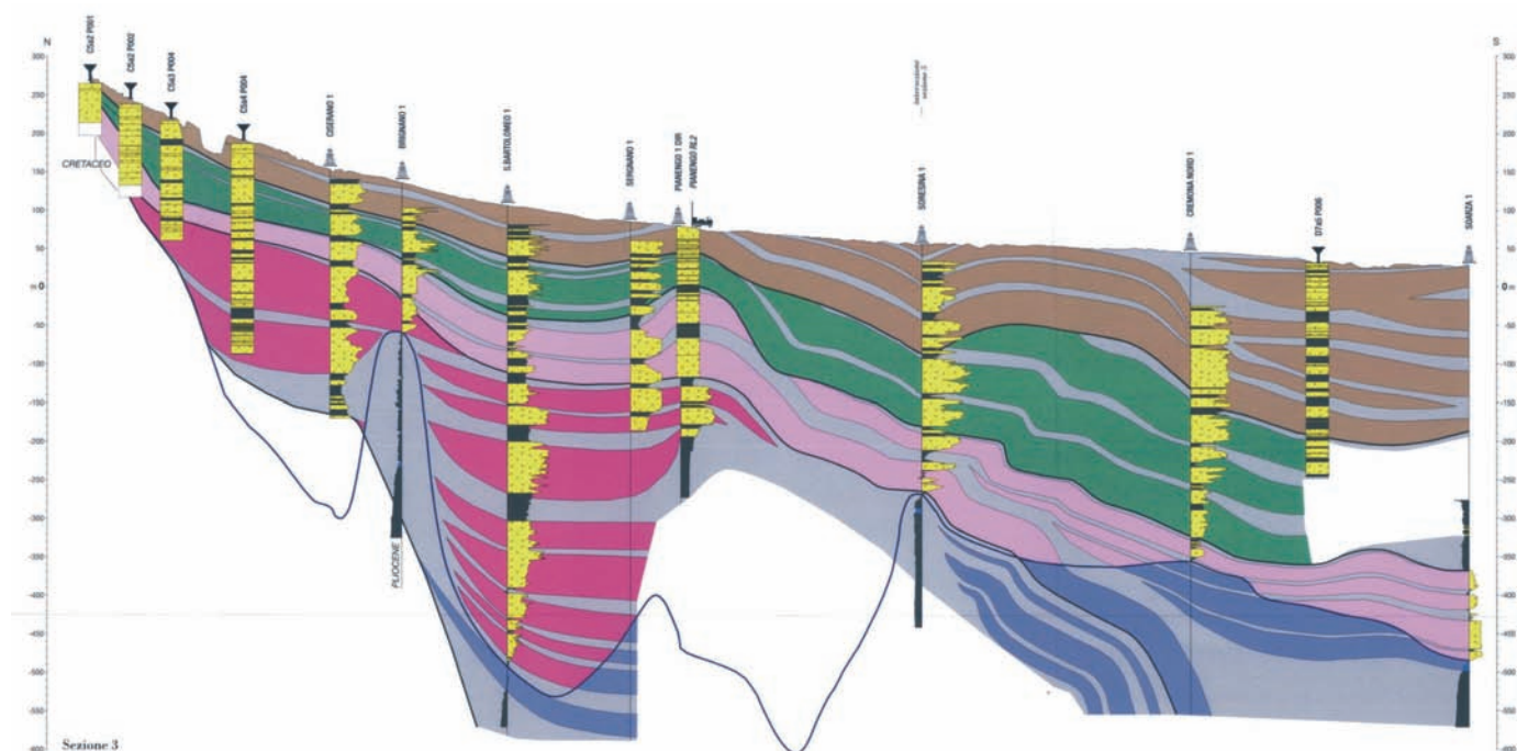
Fig. 6 - Geologia degli acquiferi padani della Regione Lombardia - Sezioni idrostratigrafiche (scala orizzontale 1:200.000, scala verticale 1:4.000) (REGIONE LOMBARDIA & ENI, 2002) - Geology of the Po River aquifers in the Lombardia Region - Hydrostratigraphic cross-sections (horizontal scale 1:200,000, vertical scale 1:4,000) (REGIONE LOMBARDIA & ENI, 2002)
